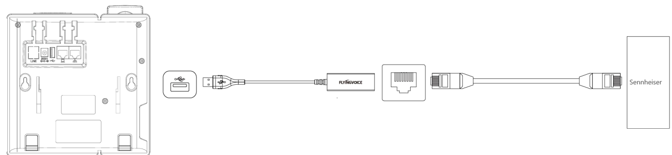
连接 Sennheiser 无线耳麦示意图
