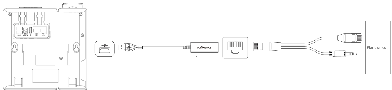
连接 Plantronics 无线耳麦示意图
